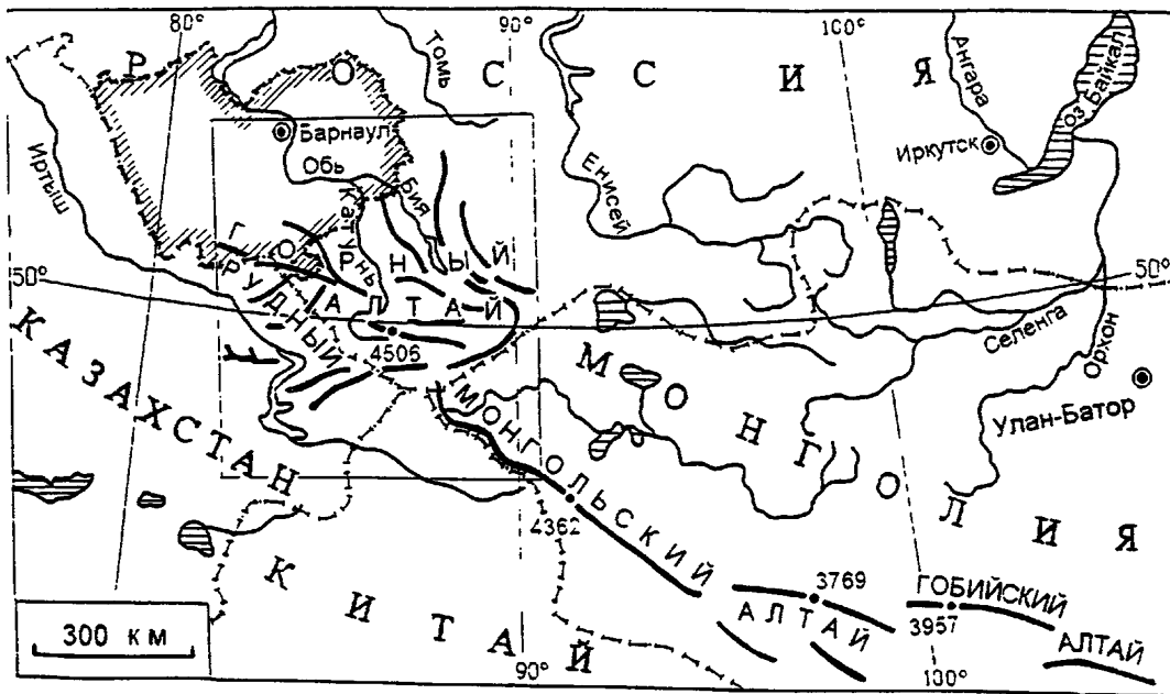
Рис. 1 Горная страна Алтай На территории России контуром обозначена современная граница Алтайского края. Выделенная рамкой территория показана на рис. 2.
