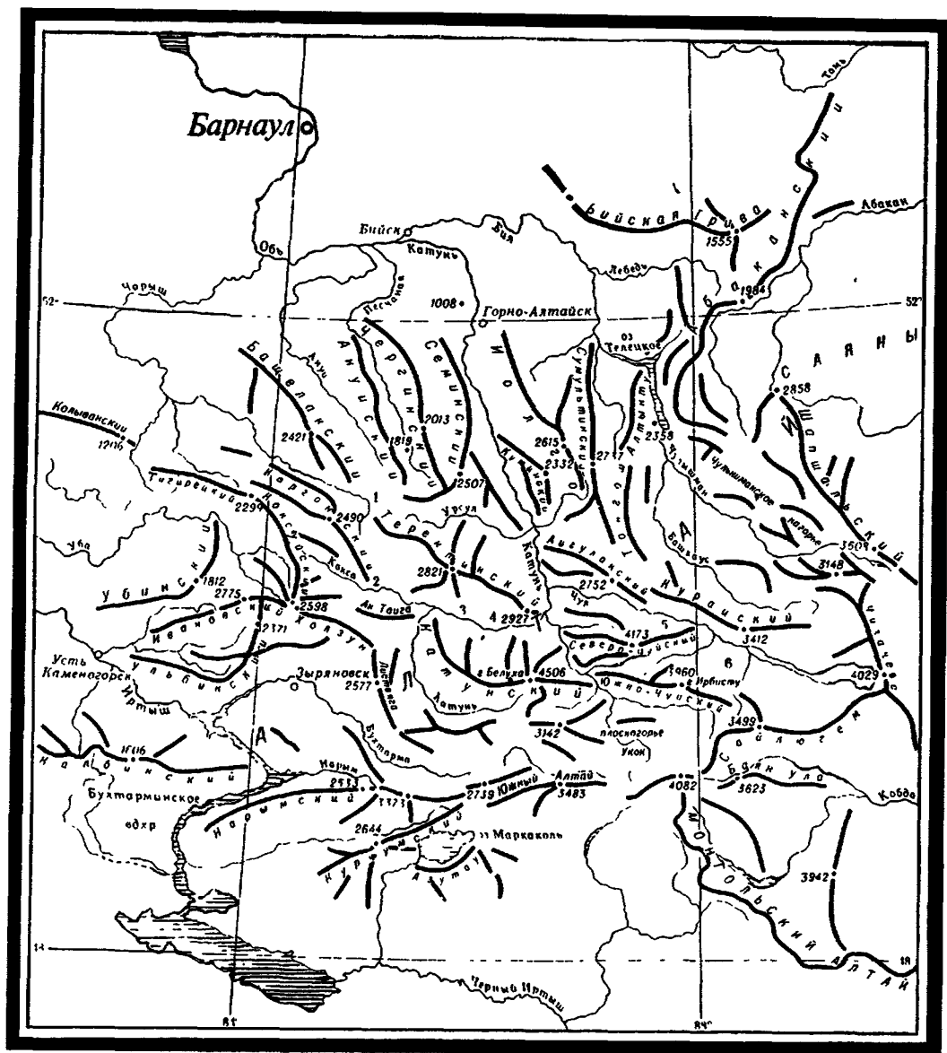
Рис. 2. Карта хребтов Горного и Рудного Алтая.
